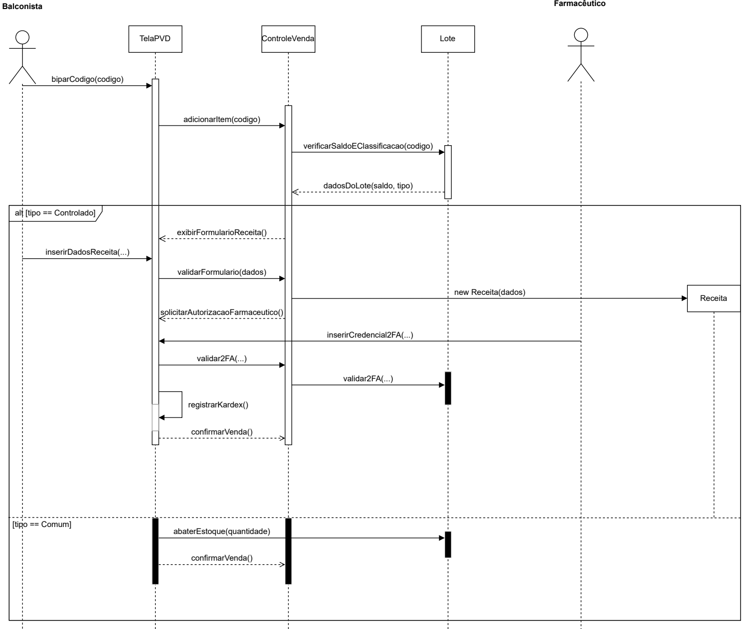
Diagrama de Sequencia Venda Controlada
